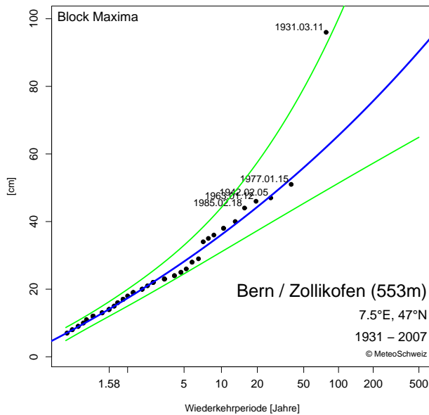
Abbildung 3.16: Gumbel-Diagramm an der Station Bern-Zollikofen für die Gesamtschneehöhe. GOF-Test: Die geschätzte Verteilung passt gut zu den Daten. Grün: 90% Konfidenzintervall.
