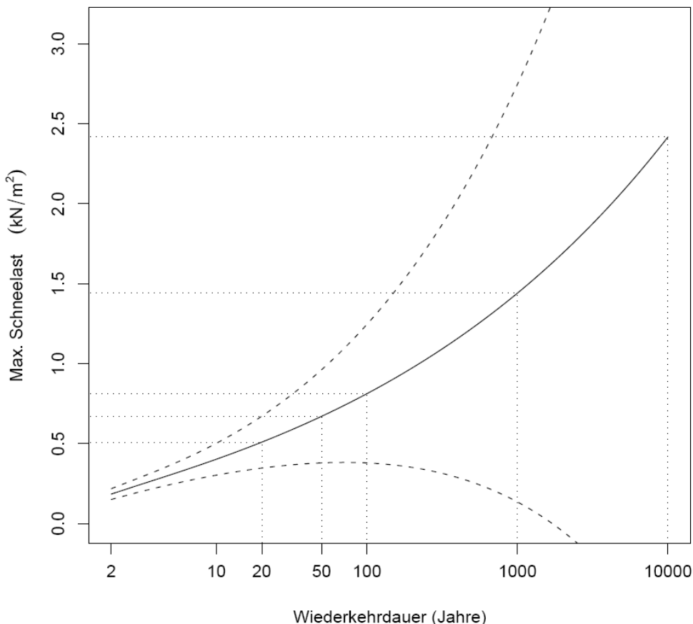
Abbildung 2.37: Extremwert-Diagramm für die Wiederkehrdauer von maximal auftretenden Schneelasten am Standort Mühleberg. Konfidenzintervalle sind nicht zuverlässig für Wiederkehrperioden die grösser sind als die zugrundeliegende Datenreihen selbst (vgl. Wiederkehrperioden > 100 Jahre). Eine Schneelast von ca. 0.81 kN/m 2 hat an der Station eine Mühleberg eine Wiederkehrperiode von 50 Jahren. Zusätzlich zeigt die obere Grenze des 95% Konfidenzintervalls, dass bei 95% der möglichen Verteilungen eine Schneelast von beispielsweise 0.81 kN/m 2 eine Wiederkehrperiode von 20 Jahren haben kann.
