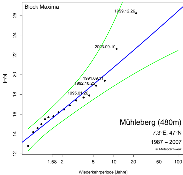
Abbildung 3.9: Gumbel-Diagramm an der Station Mühleberg für das 10-Minuten Mittel der Windgeschwindigkeit beim 110 m Messniveau. GOF-Test: die geschätzte Verteilung passt gut zu den Daten. Grün: 90% Konfidenzintervall.
