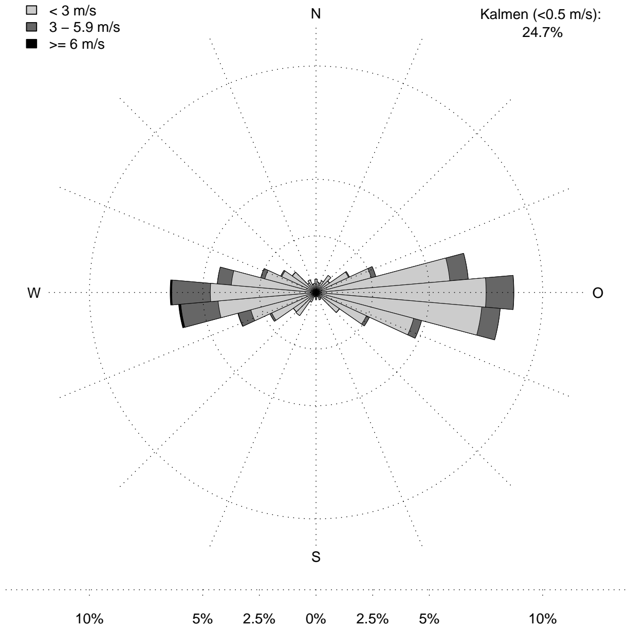
Abbildung 2.25: Mittlere jährliche Windrose der Periode 01.02.1987 bis 31.12.2007 am Standort Mühleberg auf dem Niveau 10 m über Grund auf Basis von Stundenmittelwerten. Die Grösse der Windrichtungsklassen beträgt 10 Grad. Windgeschwindigkeiten unter 0.5 m/s (Kalmen) werden nicht dargestellt.
