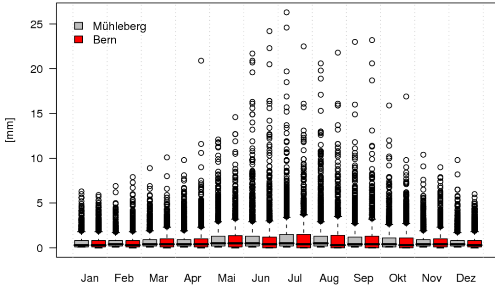
Abbildung 2.19: Vergleich der stündlichen Niederschlagssummen von Mühleberg und Bern/Liebefeld in der Periode 12.10.1988 bis 31.12.2007. Die Boxplots zeigen die Verteilung der Stundenwerte separat an beiden Stationen für jeden Monat. Stunden ohne Niederschlag wurden für die Darstellung nicht berücksichtigt. Der Aufbau der Boxplots ist analog zu Abbildung 2.13. Da Niederschlagsmengen eine schiefe Verteilung aufweisen, ist die Vergleichbarkeit der Verteilungen mit Boxplots allerdings eingeschränkt.
