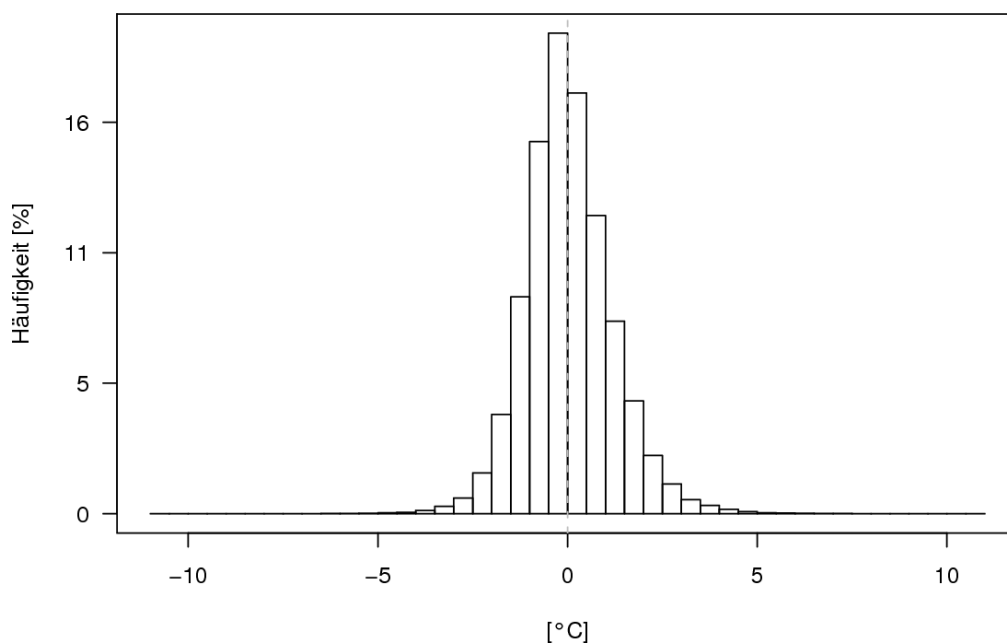
Abbildung 2.2: Häufigkeitsverteilung der Differenzen der Temperatur-Stundenmittel von Mühleberg und Wynau (Mühleberg minus Wynau) in Klassen von 0.5 Grad Celsius.
