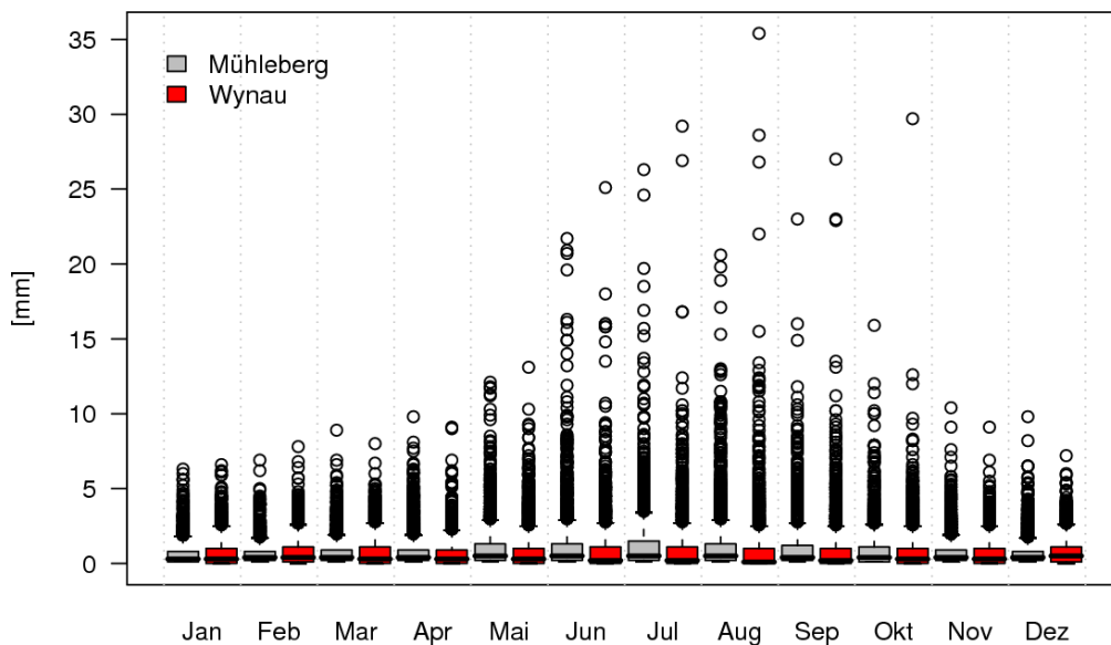
Abbildung 2.7: Vergleich der stündlichen Niederschlagssummen von Mühleberg und Wynau in der Periode 27.10.1988 bis 31.12.2007. Die Boxplots zeigen die Verteilung der Stundenwerte separat an beiden Stationen für jeden Monat. Stunden ohne Niederschlag wurden für die Darstellung nicht berücksichtigt. Der Aufbau der Boxplots ist analog zu Abbildung 2.1. Da Niederschlagsmengen eine schiefe Verteilung aufweisen, ist die Vergleichbarkeit der Verteilungen mit Boxplots allerdings eingeschränkt.
