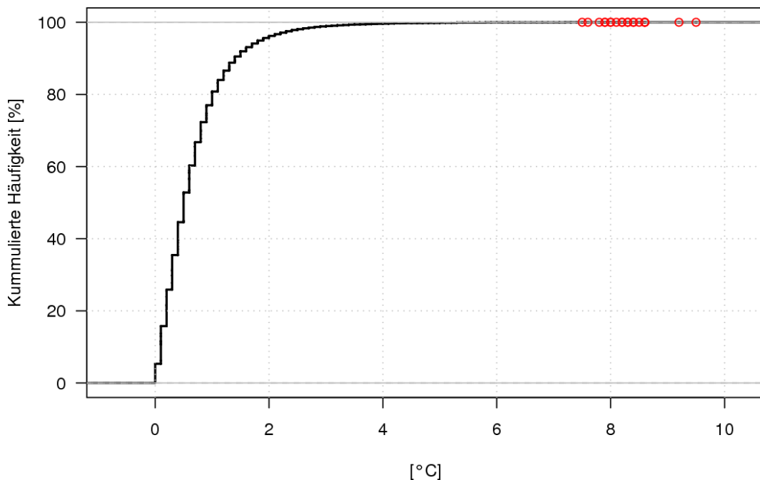
Abbildung 2.15: Kumulierte Häufigkeitsverteilung der absoluten Differenzen der Temperatur-Stundenmittel von Mühleberg und Bern/Liebefeld (Mühleberg minus Bern/Liebefeld). Es kann abgelesen werden, welcher Prozentsatz der Differenzen kleiner oder gleich einem bestimmten Wert ist. Die 20 grössten Differenzen sind mit roten Kreisen hervorgehoben.
