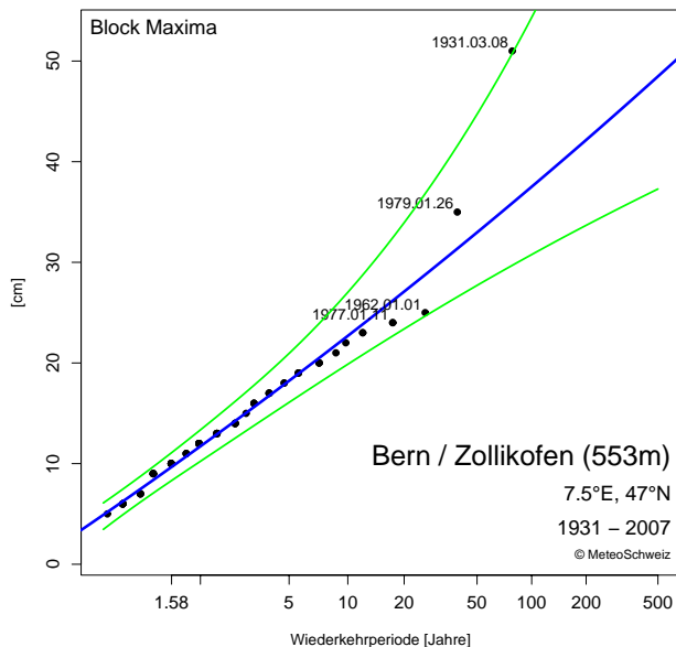
Abbildung 3.12: Gumbel-Diagramm an der Station Bern-Zollikofen für den 1-Tages Neuschnee. GOF-Test: Die geschätzte Verteilung passt gut zu den Daten. Grün: 90% Konfidenzintervall.
