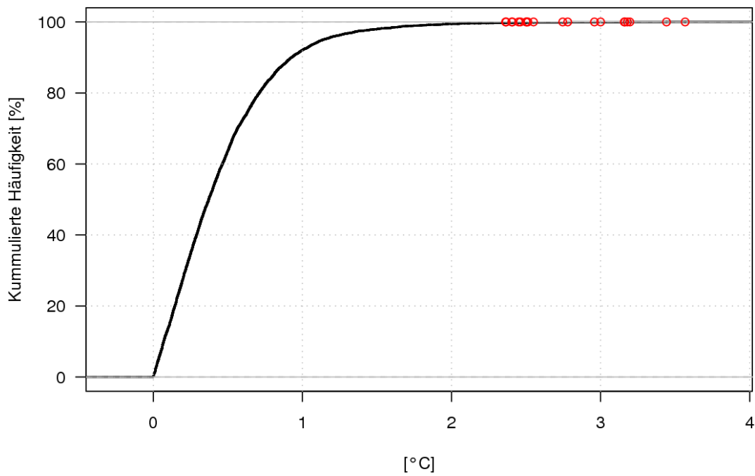
Abbildung 2.18: Gleich wie Abbildung 2.15 aber für die Tagesmittelwerte.
