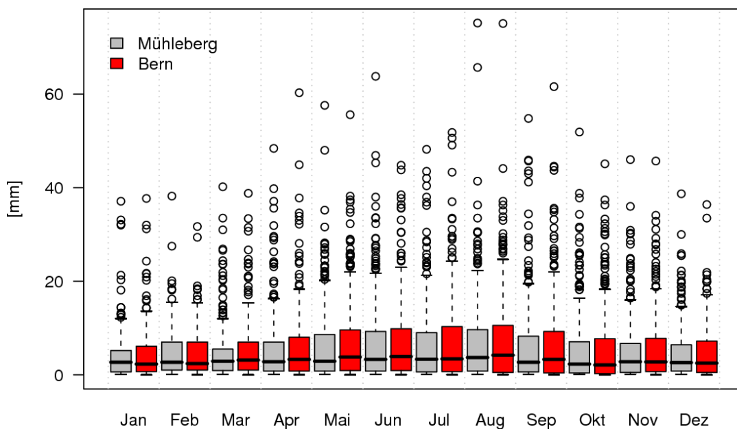
Abbildung 2.22: Gleich wie Abbildung 2.19 aber für die Tagessummen.
