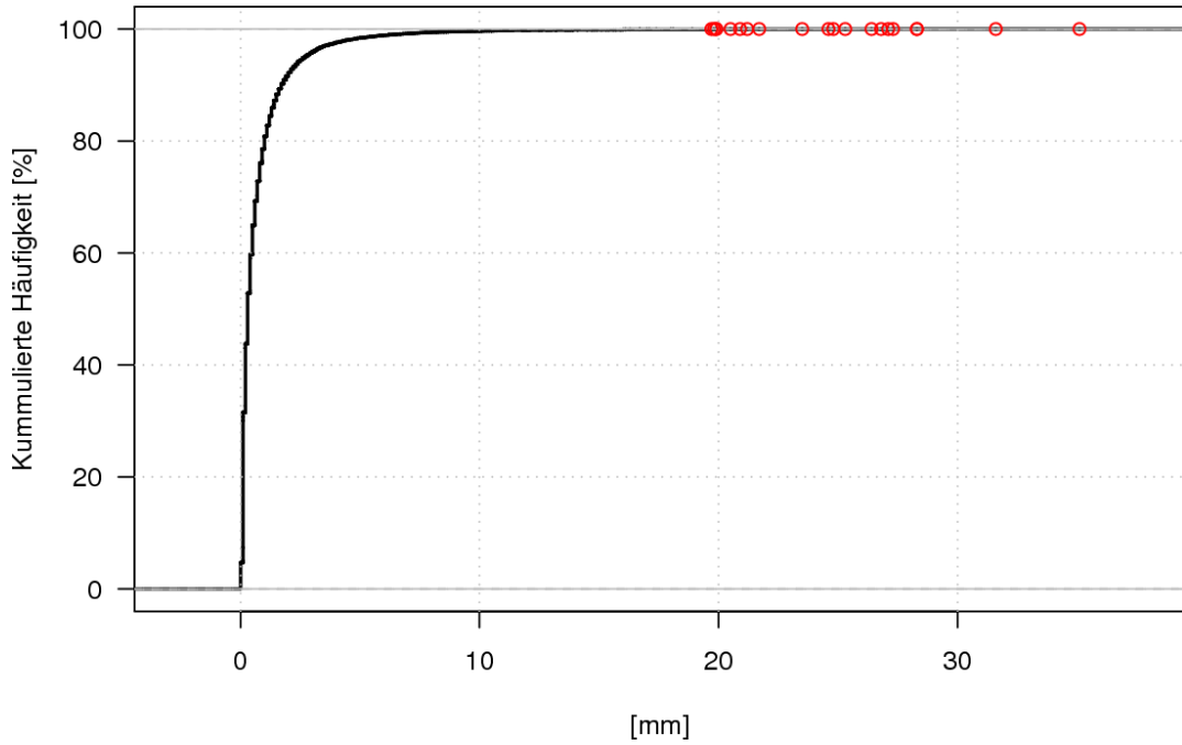
Abbildung 2.9: Kummulierte Häufigkeitsverteilung der absoluten Differenzen der stündlichen Niederschlagssummen von Mühleberg und Wynau (Mühleberg minus Wynau). Stunden, die an beiden Stationen keinen Niederschlag aufweisen, wurden für die Darstellung nicht verwendet. Es kann abgelesen werden, welcher Prozentsatz der Differenzen kleiner oder gleich einem bestimmten Wert ist. Die 20 grössten Differenzen sind mit roten Kreisen hervorgehoben.
