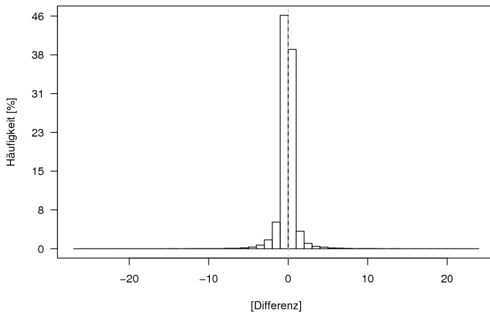
Abbildung 2.20: Häufigkeitsverteilung der Differenzen der stündlichen Niederschlagssummen von Mühleberg und Bern/Liebefeld (Mühleberg minus Bern/Liebefeld) in Klassen von 1 mm. Stunden, die an beiden Stationen keinen Niederschlag aufweisen, wurden für die Darstellung nicht verwendet.
