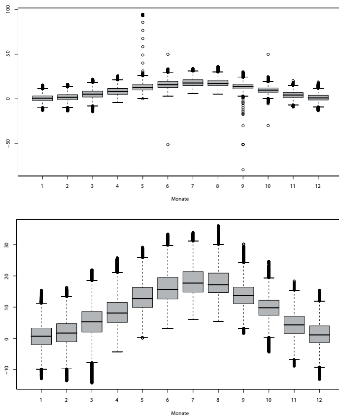
Abbildung 1.2: Temperatur Datenreihen von Mühleberg, 10 m Messniveau vor (oben) und nach (unten) der Datenbearbeitung.
