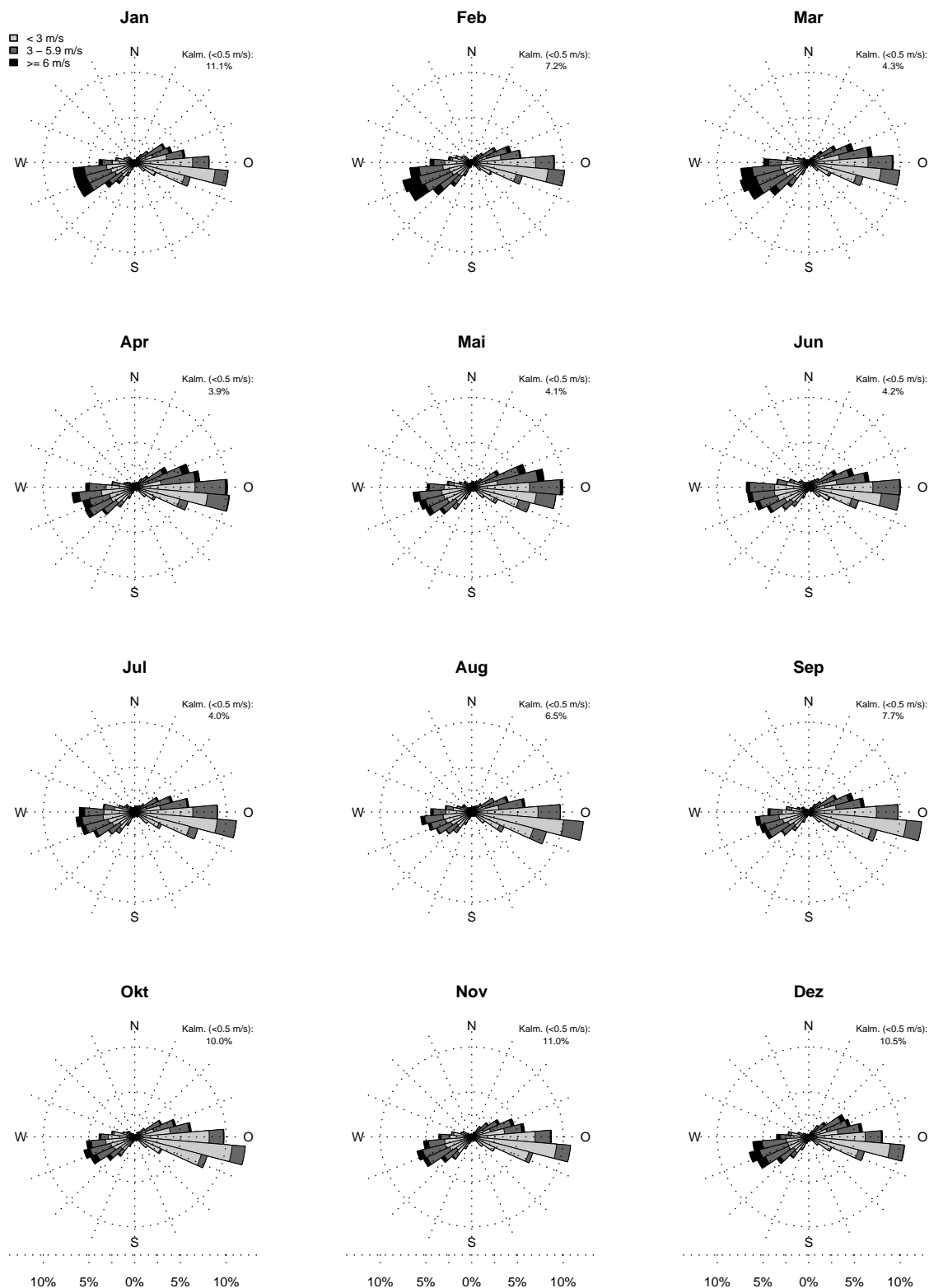
Abbildung 2.28: Mittlere monatliche Windrose der Periode 01.02.1987 bis 31.12.2007 am Standort Mühleberg auf dem Niveau 110 m über Grund auf Basis von Stundenmittelwerten. Die Grösse der Windrichtungsklassen beträgt 10 Grad. Windgeschwindigkeiten unter 0.5 m/s (Kalmen) werden nicht dargestellt.
