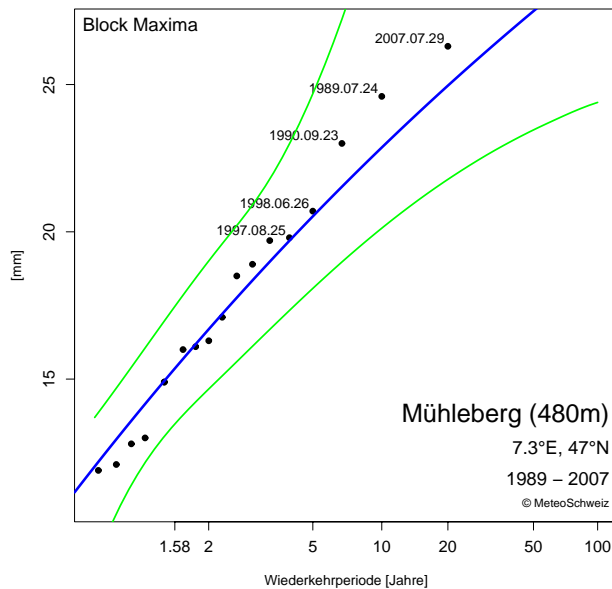
Abbildung 3.1: Gumbel-Diagramm an der Station Mühleberg für den stündlichen Niederschlag. GOF-Test: Da der GOF-Test nicht durchgeführt werden konnte, gibt es keine Angaben zur Güte des Fits. Grün: 90% Konfidenzintervall.
