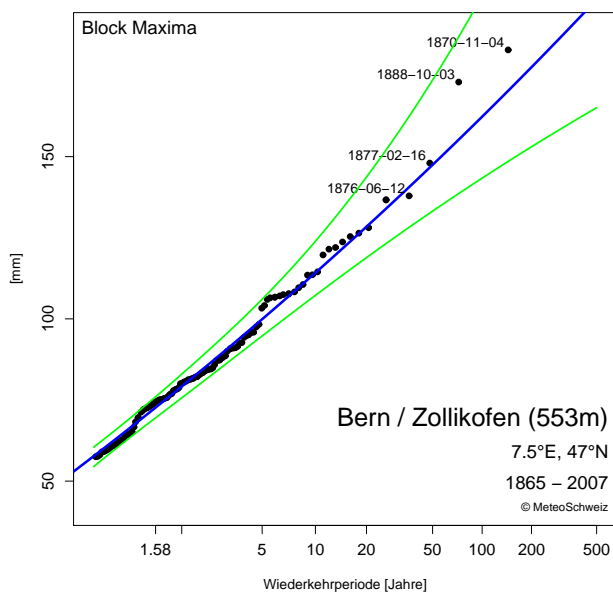
Abbildung 3.4: Gumbel-Diagramm an der Station Bern/Zollikofen für den 5-Tages Niederschlag. GOF-Test: Die geschätzte Verteilung passt gut zu den Daten. Grün: 90% Konfidenzintervall.
