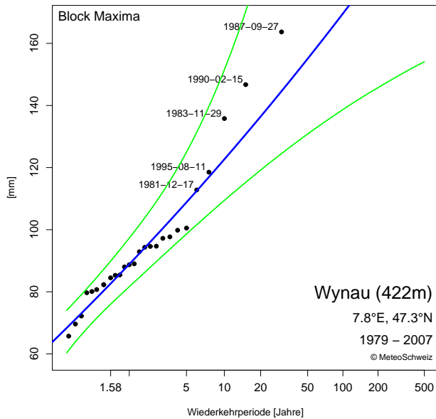
Abbildung 3.5: Gumbel-Diagramm an der Station Wynau für den 5-Tages Niederschlag. GOF-Test: Die geschätzte Verteilung passt nicht gut zu den Daten. Grün: 90% Konfidenzintervall.
