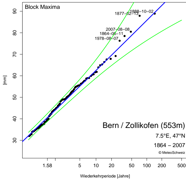
Abbildung 3.2: Gumbel-Diagramm an der Station Bern/Zollikofen für den 1-Tages Niederschlag. GOF-Test: Die geschätzte Verteilung passt gut zu den Daten. Aus Datenqualitätsgründen wurde das Jahr 1870 ausgelassen. Grün: 90% Konfidenzintervall.
