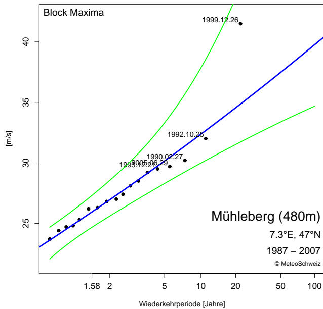
Abbildung 3.7: Gumbel-Diagramm an der Station Mühleberg für die 10-Minuten Böenspitze 110 m über Grund. GOF-Test: die geschätzte Verteilung passt gut zu den Daten. Grün: 90% Konfidenzintervall.
