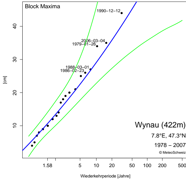
Abbildung 3.13: Gumbel-Diagramm an der Station Wynau für den 1-Tages Neuschnee. GOF-Test: Die geschätzte Verteilung passt gut zu den Daten. Grün: 90% Konfidenzintervall.
