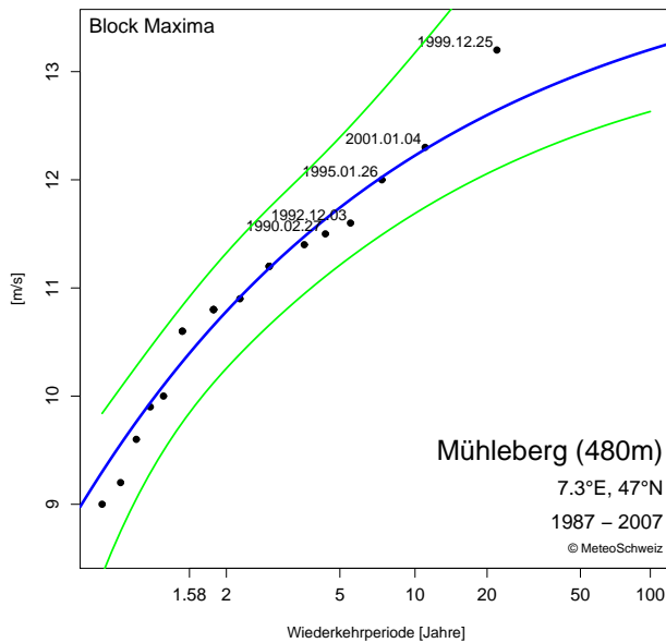
Abbildung 3.8: Gumbel-Diagramm an der Station Mühleberg für das 10-Minuten Mittel der Windgeschwindigkeit, 10 m über Grund. GOF-Test: Da der GOF-Test nicht durchgeführt werden konnte, gibt es keine Angaben zur Güte des Fits. Grün: 90% Konfidenzintervall.
