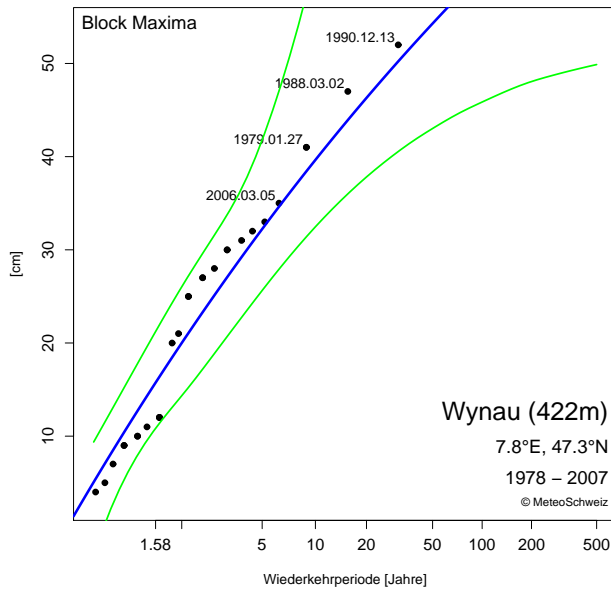
Abbildung 3.17: Gumbel-Diagramm an der Station Wynau für die Gesamtschneehöhe. GOF-Test: Die geschätzte Verteilung passt nicht gut zu den Daten. Grün: 90% Konfidenzintervall.
