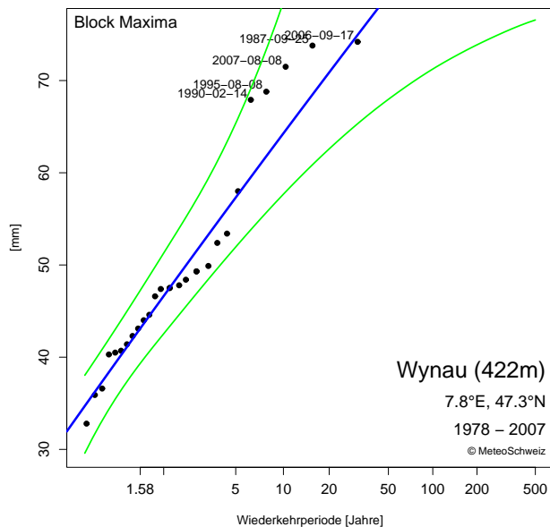
Abbildung 3.3: Gumbel-Diagramm an der Station Wynau für den 1-Tages Niederschlag. GOF-Test: Die geschätzte Verteilung passt gut zu den Daten. Grün: 90% Konfidenzintervall.
