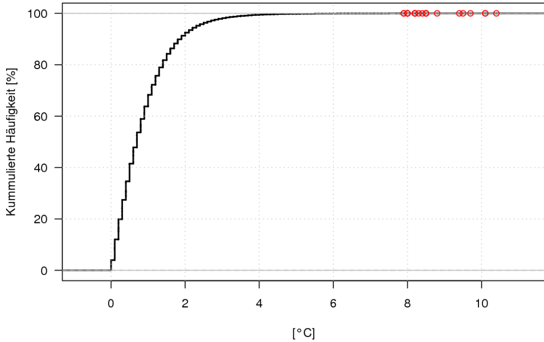
Abbildung 2.3: Kumulierte Häufigkeitsverteilung der absoluten Differenzen der Temperatur-Stundenmittel von Mühleberg und Wynau (Mühleberg minus Wynau). Es kann abgelesen werden, welcher Prozentsatz der Differenzen kleiner oder gleich einem bestimmten Wert ist. Die 20 grössten Differenzen sind mit roten Kreisen hervorgehoben.
