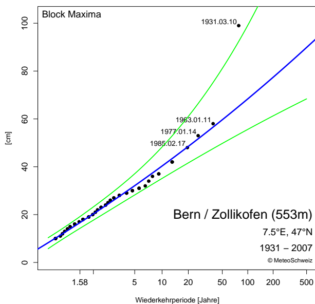
Abbildung 3.14: Gumbel-Diagramm an der Station Bern-Zollikofen für den 5-Tages Neuschnee. GOF-Test: Die geschätzte Verteilung passt gut zu den Daten. Grün: 90% Konfidenzintervall.
