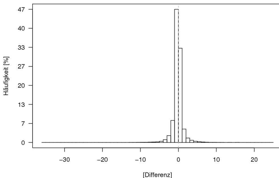
Abbildung 2.8: Häufigkeitsverteilung der Differenzen der stündlichen Niederschlagssummen von Mühleberg und Wynau (Mühleberg minus Wynau) in Klassen von 1 mm. Stunden, die an beiden Stationen keinen Niederschlag aufweisen, wurden für die Darstellung nicht verwendet.
