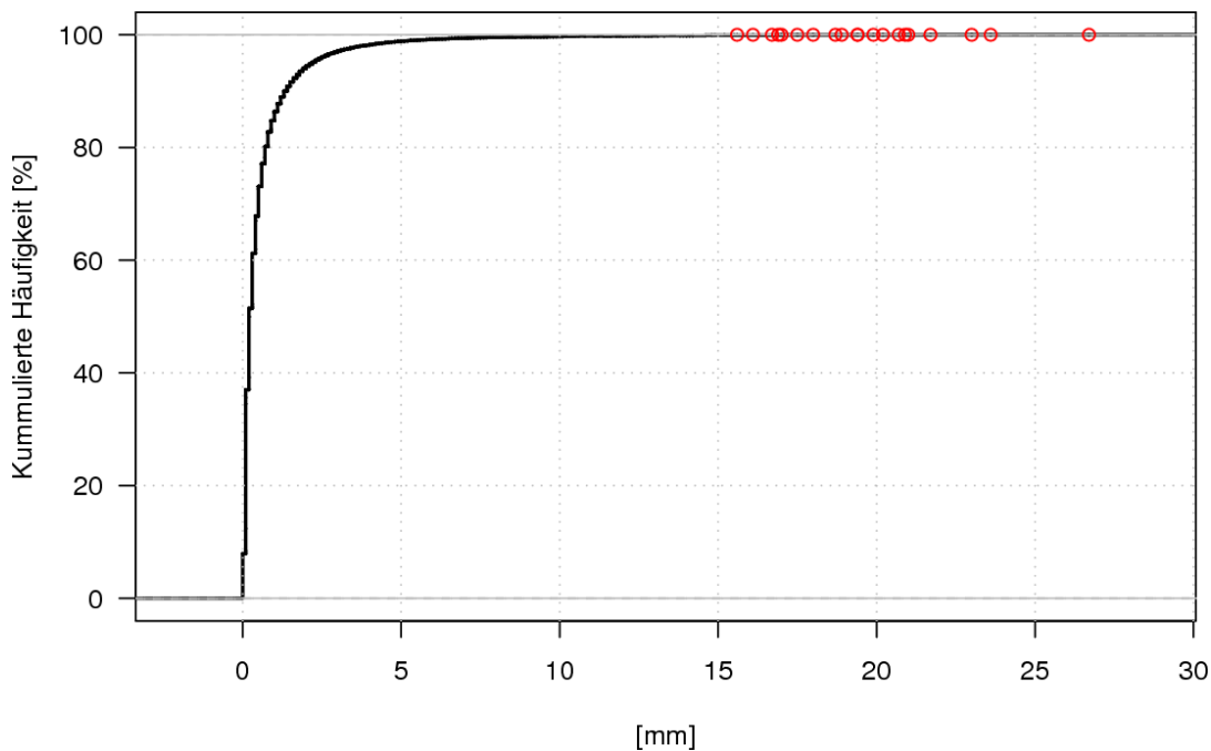
Abbildung 2.21: Kummulierte Häufigkeitsverteilung der absoluten Differenzen der stündlichen Niederschlagssummen von Mühleberg und Bern/Liebefeld (Mühleberg minus Bern/Liebefeld). Stunden, die an beiden Stationen keinen Niederschlag aufweisen, wurden für die Darstellung nicht verwendet. Es kann abgelesen werden, welcher Prozentsatz der Differenzen kleiner oder gleich einem bestimmten Wert ist. Die 20 grössten Differenzen sind mit roten Kreisen hervorgehoben.
