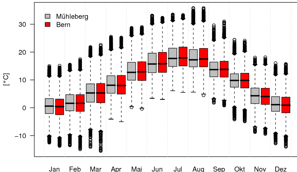
Abbildung 2.13: Vergleich der stündlichen Temperaturmittel von Mühleberg und Bern/Liebefeld in der Periode 1.2.1987 bis 31.12.2007. Die Boxplots zeigen die Verteilung der Stundenwerte separat an beiden Stationen für jeden Monat. Die Box der Boxplots umfasst die Messwerte zwischen dem 25%- und dem 75%-Quantil. Der Median wird durch eine Linie repräsentiert. Die sog. Whiskers (gestrichelte Linien) decken 1.5-mal die Box-Spannbreite gegen oben und unten ab und zeigen den Wertebereich der meisten Stundenwerte im entsprechenden Monat. Werte ausserhalb dieser Spannbreite können als Extremwerte bezeichnet werden und sind als Punkte einzeln dargestellt.
