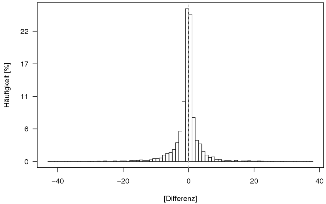
Abbildung 2.23: Gleich wie Abbildung 2.20 aber für die Tagessummen.
