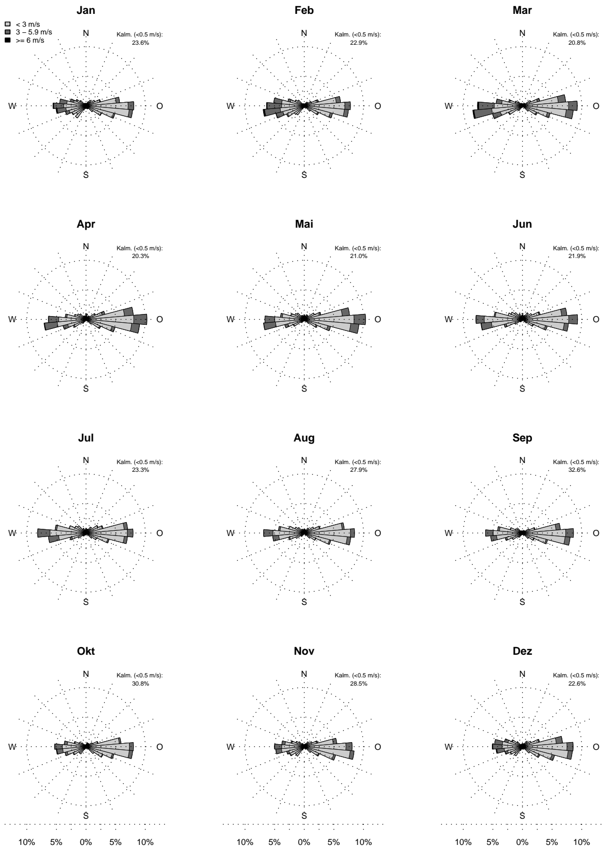
Abbildung 2.26: Mittlere monatliche Windrose der Periode 01.02.1987 bis 31.12.2007 am Standort Mühleberg auf dem Niveau 10 m über Grund auf Basis von Stundenmittelwerten. Die Grösse der Windrichtungsklassen beträgt 10 Grad. Windgeschwindigkeiten unter 0.5 m/s (Kalmen) werden nicht dargestellt.
