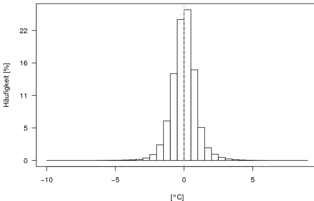
Abbildung 2.14: Häufigkeitsverteilung der Differenzen der Temperatur-Stundenmittel von Mühleberg und Bern/Liebefeld (Mühleberg minus Bern/Liebefeld) in Klassen von 0.5 Grad Celsius.
