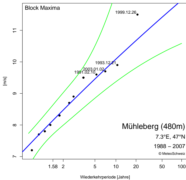
Abbildung 3.10: Gumbel-Diagramm an der Station Mühleberg für das Stundenmittel der Windgeschwindigkeit, 10 m über Grund. GOF-Test: Die geschätzte Verteilung passt gut zu den Daten. Grün: 90% Konfidenzintervall. Sturm Lothar (26.12.1999) ist klar erkennbar.
