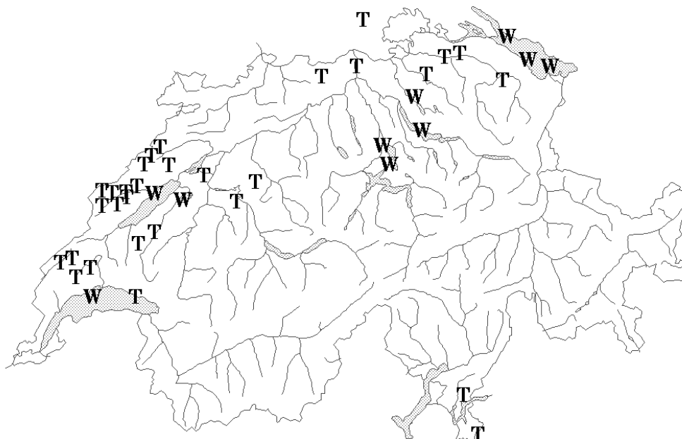
Abbildung 2.38: Registrierte Tornados (T) in der Schweiz. Mit W sind registrierte Tornados über Wasserflächen festgehalten, welche im Volksmund oft als „Wasserhosen“ bezeichnet werden. Daten: ETH Zürich, 2001, ergänzt mit Beobachtungen bis 2005.
