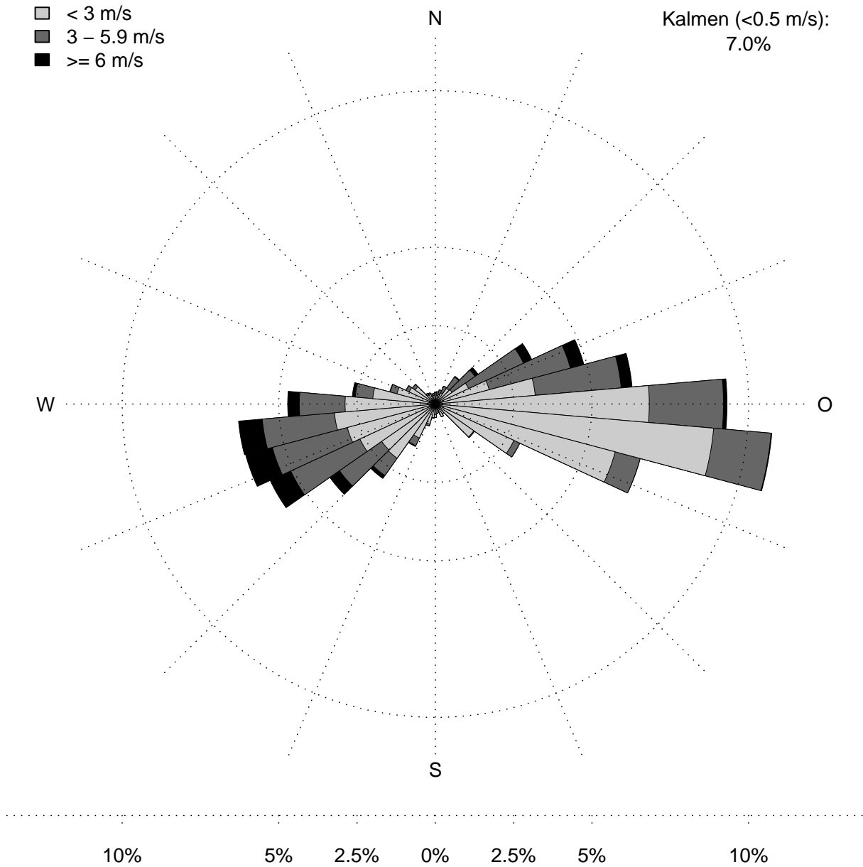
Abbildung 2.27: Mittlere jährliche Windrose der Periode 01.02.1987 bis 31.12.2007 am Standort Mühleberg auf dem Niveau 110 m über Grund auf Basis von Stundenmittelwerten. Die Grösse der Windrichtungsklassen beträgt 10 Grad. Windgeschwindigkeiten unter 0.5 m/s (Kalmen) werden nicht dargestellt.
