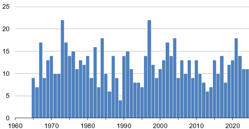
Figure 5. Nombre de jours avec du gel au sol (température minimale journalière à 5 cm au-dessus de l'herbe < 0 °C) en avril sur la période 1965-2024, moyenné pour les stations de Genève/Cointrin, Payerne et Zurich-Kloten.
