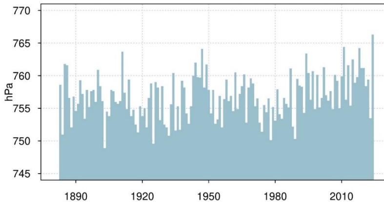
Figure 3. Pression atmosphérique maximale au mois d'avril sur le Säntis depuis le début des mesures en 1883.
