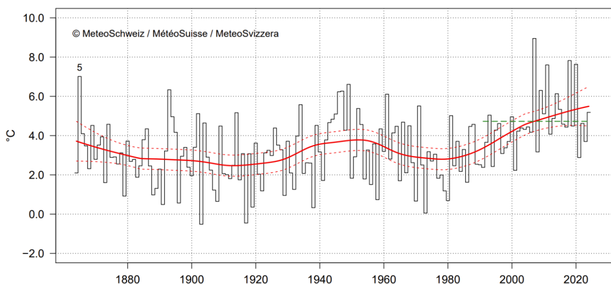
Figure 1. La température en avril en Suisse depuis le début des mesures en 1864. Elle a atteint 5,2 °C, soit 0,5 °C au-dessus de la norme 1991-2020 (ligne verte en traitillé). La ligne rouge indique la tendance climatique. Les lignes rouges en traitillé montrent l'incertitude de la tendance climatique.
