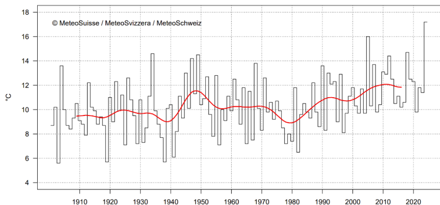
Figure 2. Période de trois jours la plus chaude du mois d'avril à La Chaux-de-Fonds depuis le début des mesures en 1901. La ligne rouge indique la moyenne glissante sur 20 ans.
