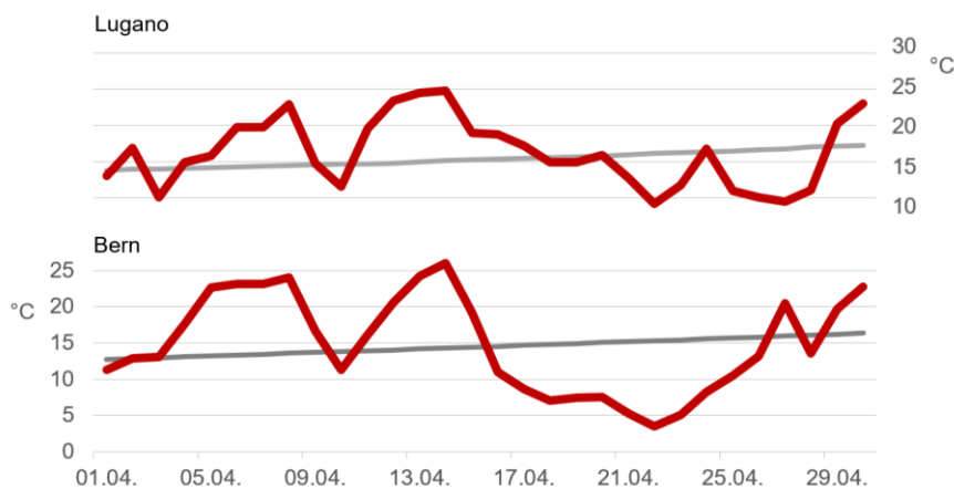
Figure 4. Evolution de la température maximale journalière en avril 2024 sur les sites de Lugano et de Berne-Zollikofen. Les lignes grises indiquent la norme 1991-2020.
