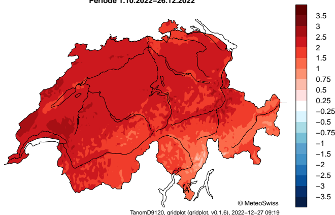
Déviations de température à 1991–2020 [°C] Période 1.10.2022–26.12.2022
