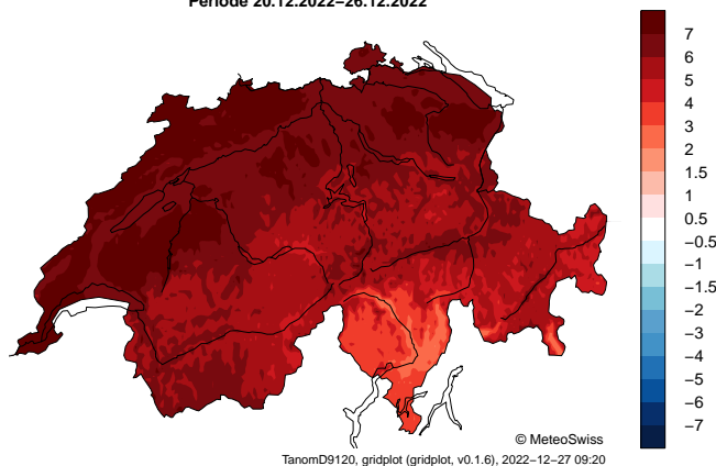
Déviations de température à 1991–2020 [°C] Période 20.12.2022–26.12.2022
